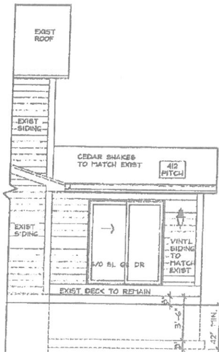
RIGHT ELEVATION
